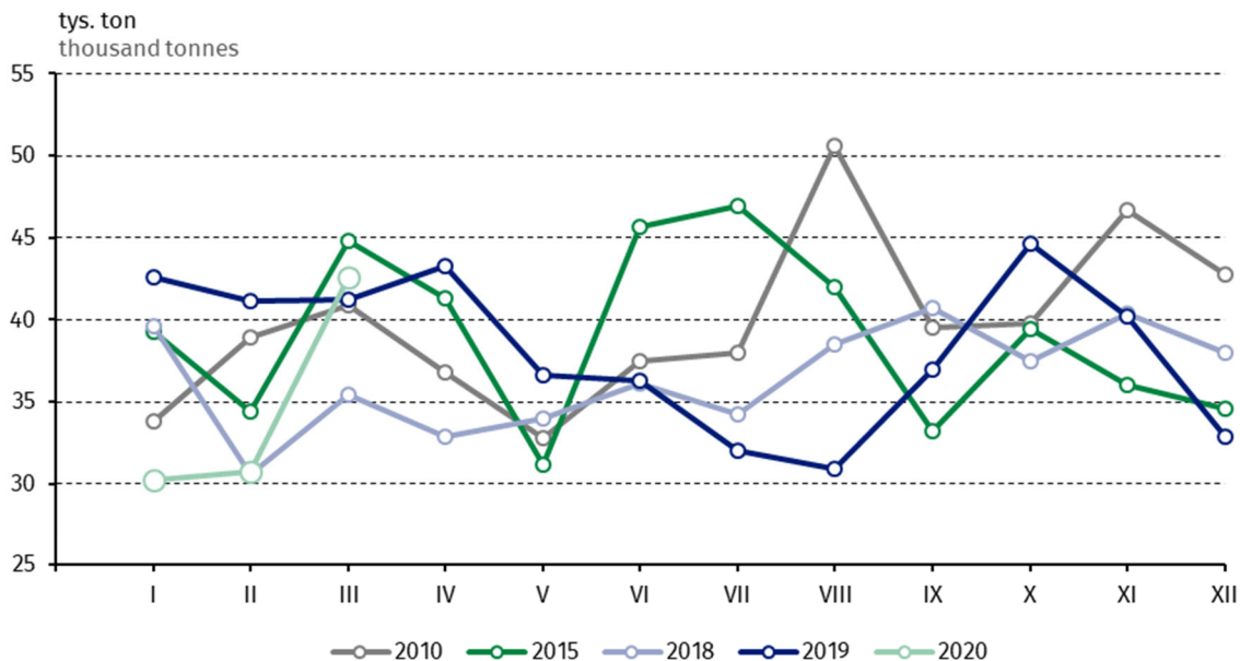
Wykres 15. Produkcja nawozów fosforowych a Chart 15. Production of phosphatic fertilizers a
