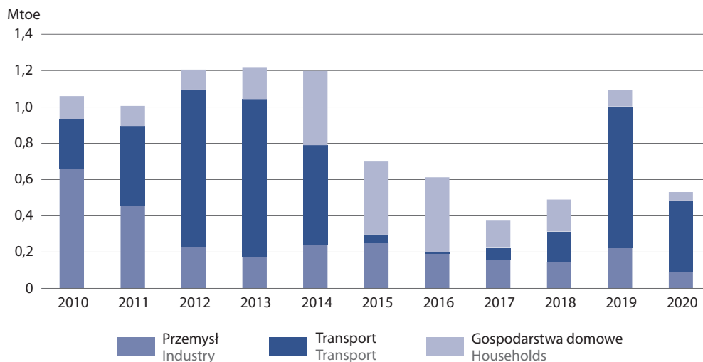
Wykres 25. Oszczędności energii wg sektorów Chart 25. Energy savings by sector
