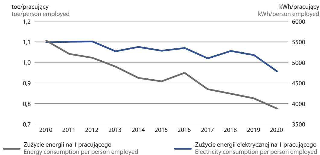
Wykres 22. Zużycie energii i energii elektrycznej w przeliczeniu na 1 pracującego w sektorze usług Chart 22. Energy and electricity consumption per person employed of the service sector
