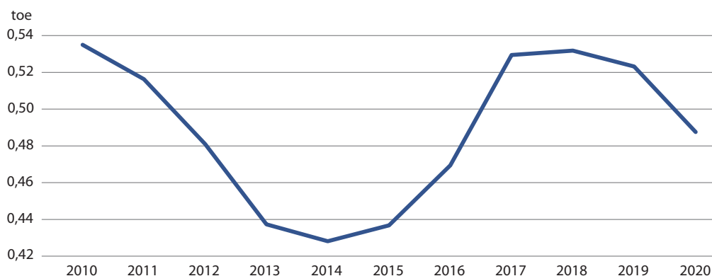
Wykres 20. Zużycie paliw przez samochód ekwiwalentny Chart 20. Fuel consumption per equivalent car
