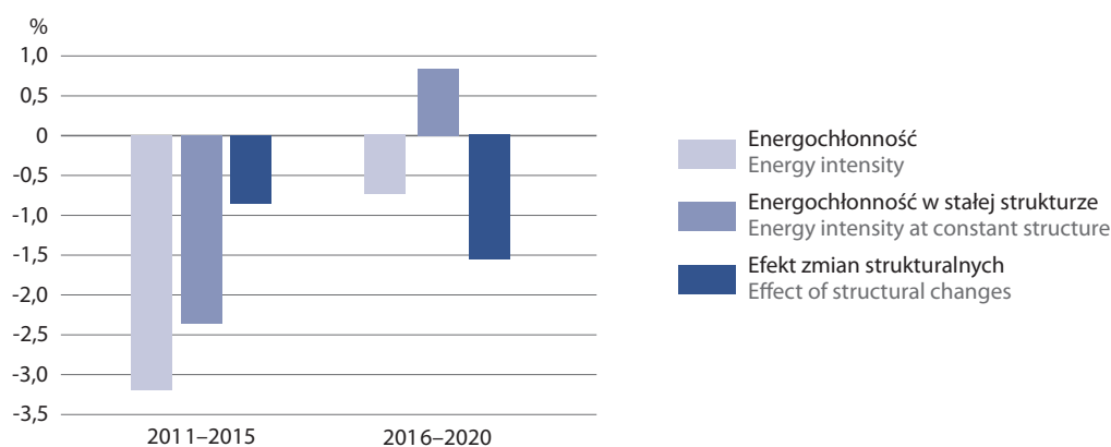
Wykres 14. Energochłonność przemysłu przetwórczego – rola zmian strukturalnych Chart 14. Energy intensity of manufacturing – role of structural changes
