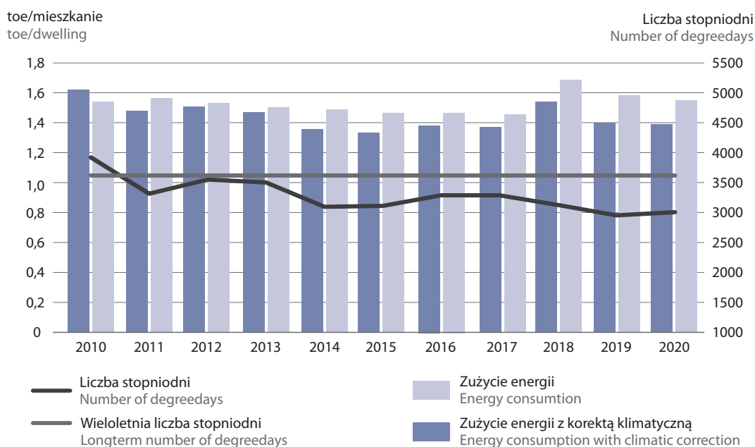
Wykres 16. Zużycie energii w gospodarstwach domowych w przeliczeniu na 1 mieszkanie Chart 16. Energy consumption in households per dwelling
