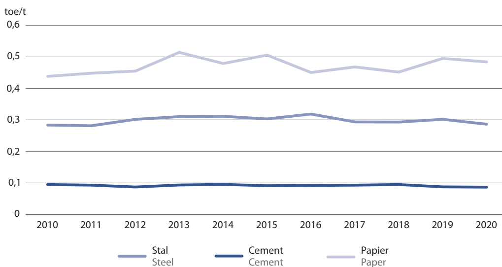
Wykres 11. Energochłonności produkcji wybranych wyrobów przemysłowych Chart 11. Unit consumption of selected industrial products
